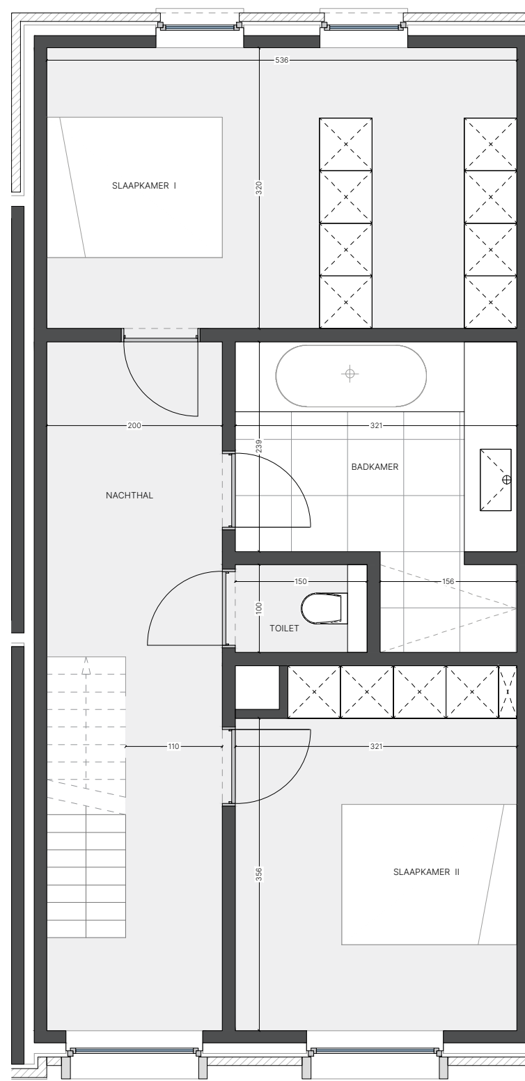
VERDIEPING +1
